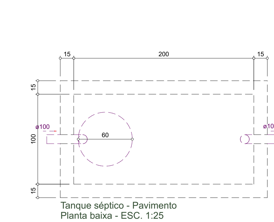
Tanque séptico - Pavimento Planta baixa - ESC. 1:25
