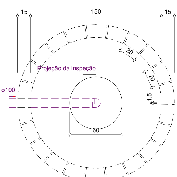
Sumidouro - Pavimento Planta baixa - ESC. 1:25
